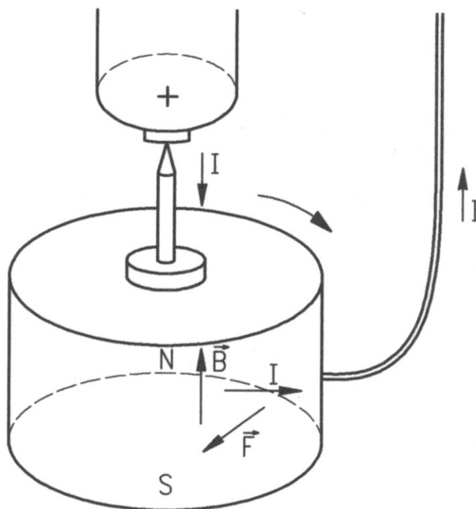
Rys. 2. Wyjaśnienie zasady działania silnika z wirującym magnesem;
