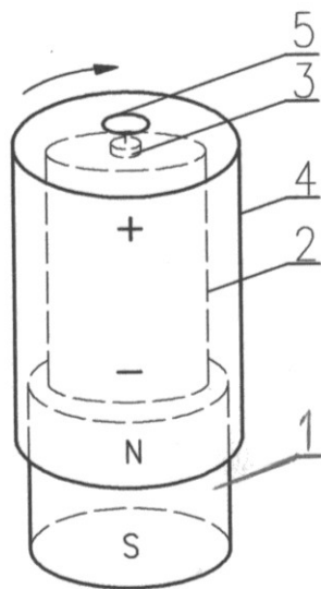
Rys. 7. Wygląd zewnętrzny silnika z obracającą się puszką; 1 – magnes neodymowy, 2 – bateria okrągła, 3 – dodatni biegun baterii, 4 – puszkę aluminiowa, 5 – pinezka.
