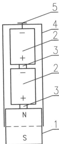
Rys. 9. Przekrój poprzeczny przez złożony silnik z obracającą się puszką, oznaczenia elementów takie same, jak w opisie rys. 7.
