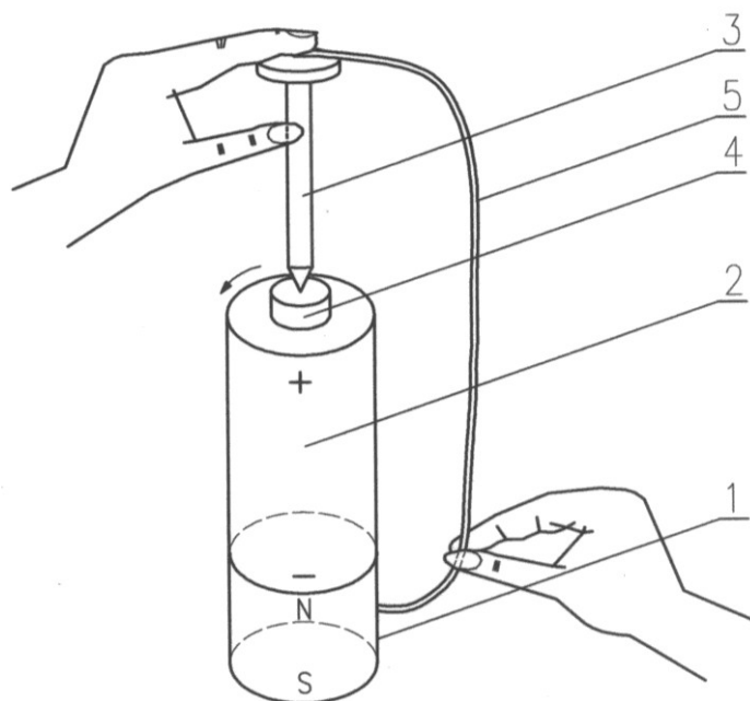
Rys. 3. Budowa silnika z wirującą baterią; 1 – magnes neodymowy, 2 – bateria typu R6, 3 – gwóźdź stalowy, 4 – dodatni biegun baterii, 5 – giętki przewód.
