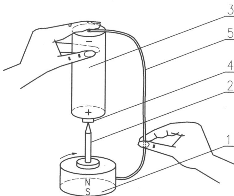
Rys. 1. Budowa silnika z wirującym magnesem; 1 – magnes neodymowy, 2 – gwóźdź stalowy, 3 – bateria typu R6, 4 – dodatni biegun baterii, 5 – giętki przewód
