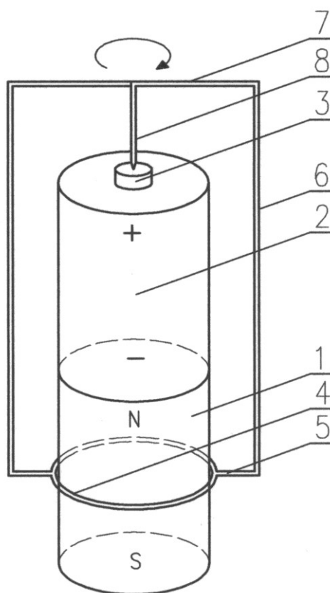
Rys. 4. Budowa silnika z wirującą ramką; 1 – magnes neodymowy, 2 – bateria typu R6, 3 – dodatni biegun baterii, 4 – pierścień ramki, 5 – dolny odcinek ramki, 6 – pionowy odcinek ramki, 7 – górny odcinek ramki, 8 – zaokrąglony koniec ramki.
